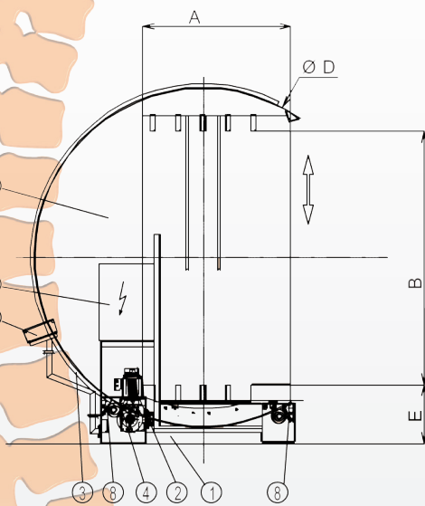
180° Wender Mit Klemmeinrichtung
